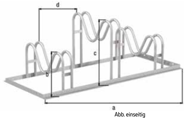
Abb. einseitig
