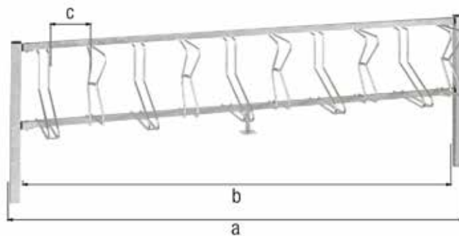
Abb. Grundelement
