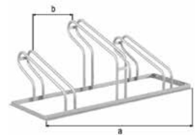
Abb. einseitig
